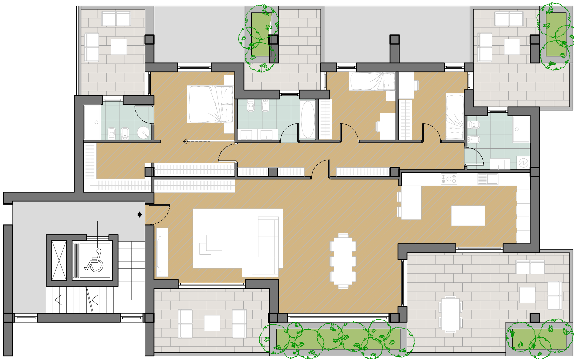
PIANO QUARTO - APPARTAMENTO "O" QUADRILOCALE MQ 180.00 TERRAZZI MQ 73.20
