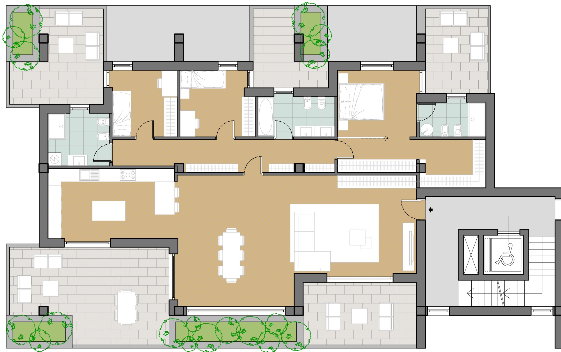
PIANO QUARTO - APPARTAMENTO "N" QUADRILOCALE MQ 180.00 TERRAZZI MQ 73.20
