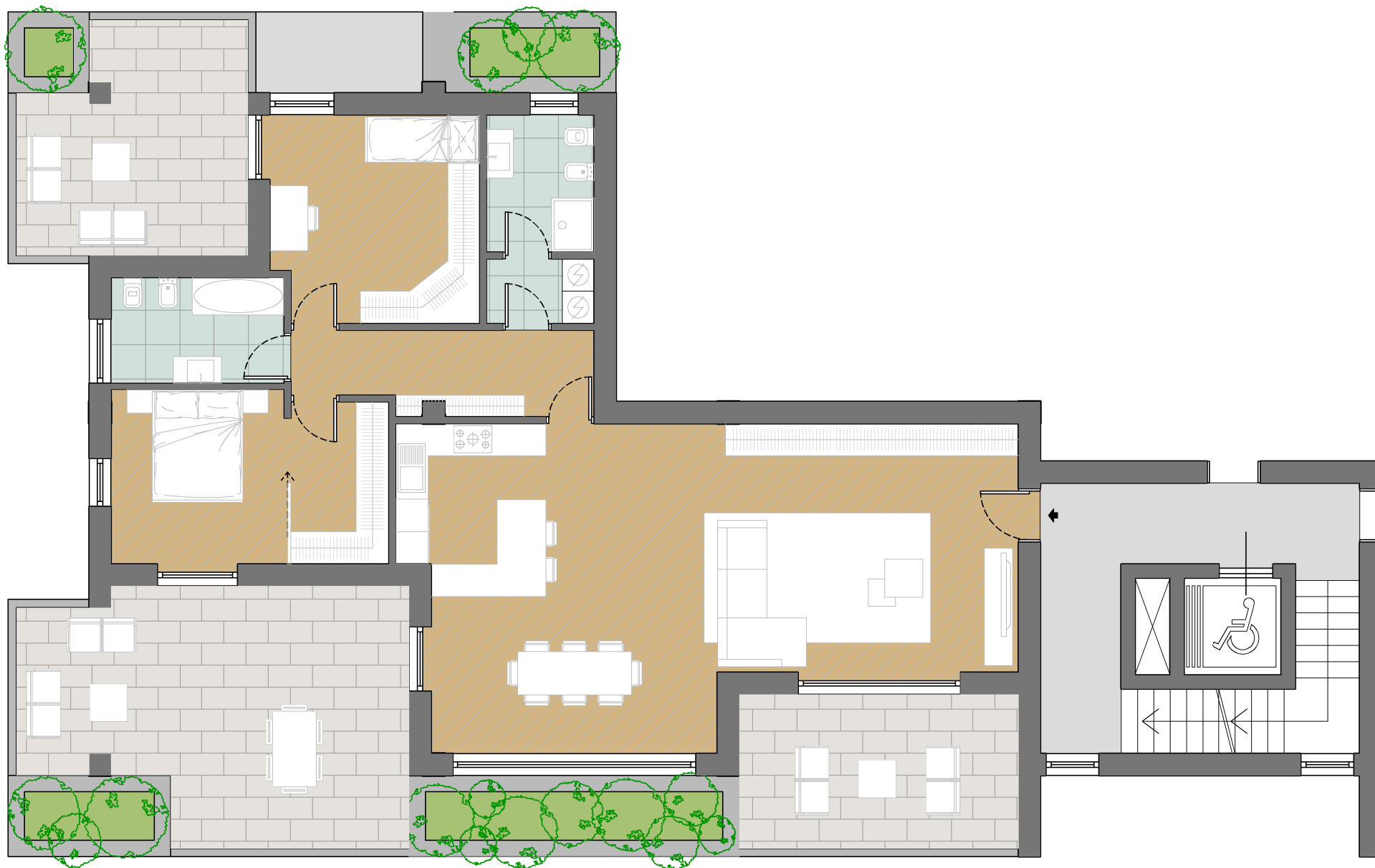
PIANO TERZO - APPARTAMENTO "I" TRILOCALE MQ 135.57 TERRAZZI MQ 65.60
