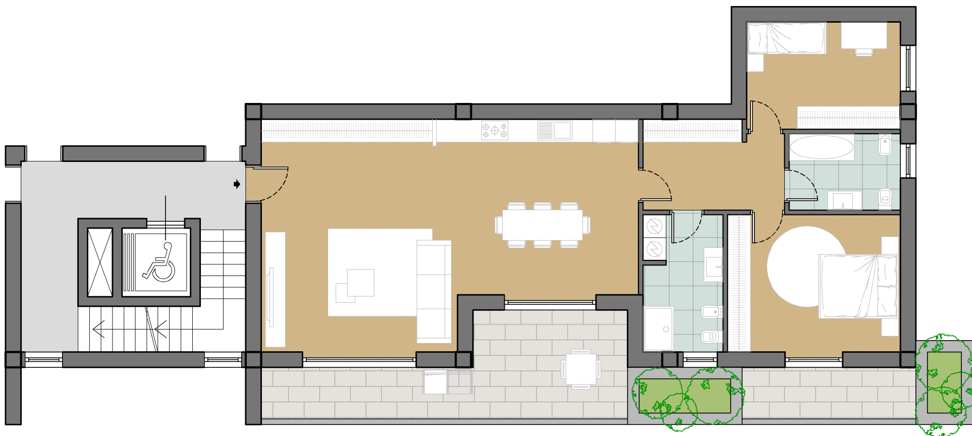
PIANO SECONDO - APPARTAMENTO "H" TRILOCALE MQ 122.84 TERRAZZI MQ 27.91
